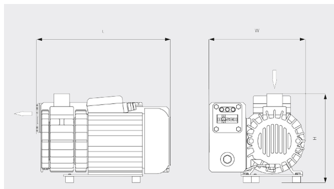
Dessin d'encombrement
